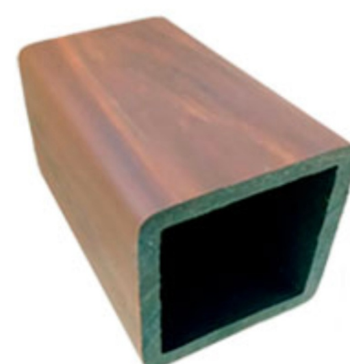
Coluna 120x120mm PESO: 5,05 Kg/m
